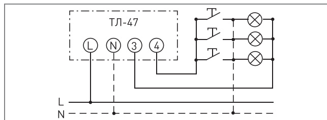
Положение переключателя 4
