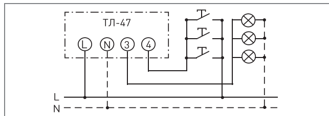
Положение переключателя 4
